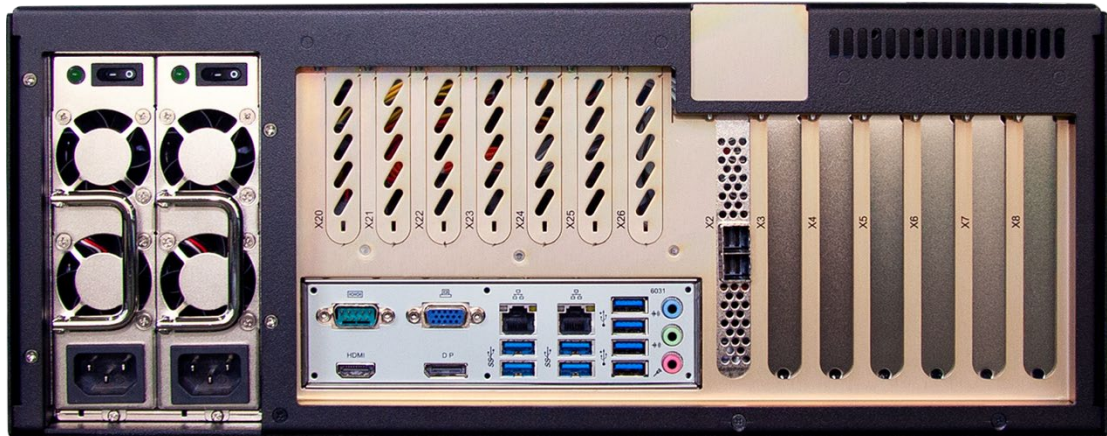
Rückansicht ibaRackline-PC CAM/HD
