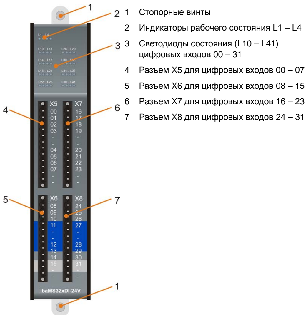
Рис. 1: Вид спереди
