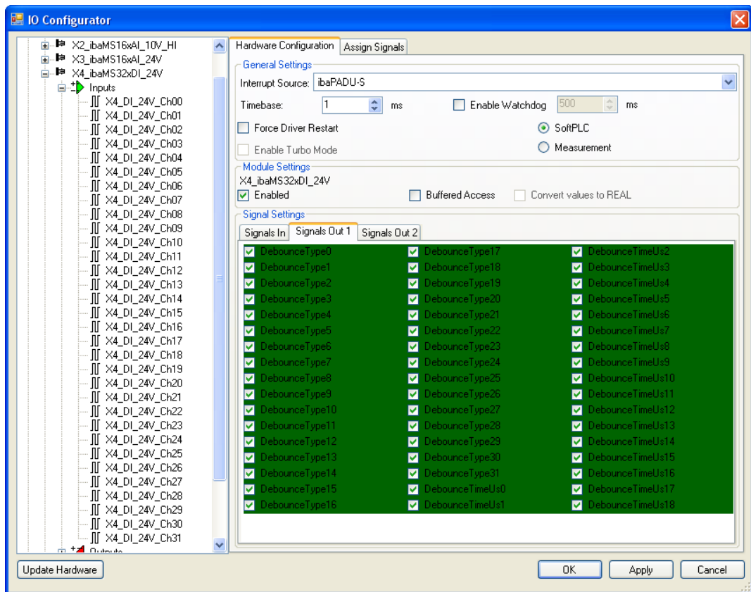
Рис. 15: Выходы ibaMS32xDI-24V
