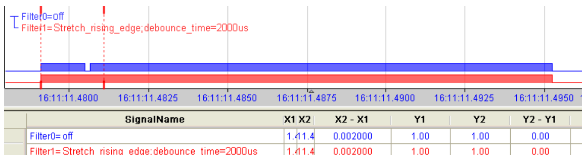
Рис. 3: Фильтр дребезга: "Растянуть передний фронт"
