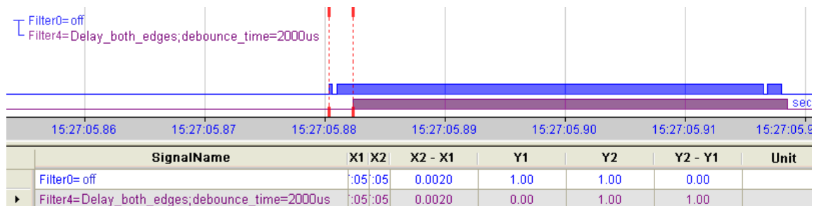
Рис. 6: Фильтр дребезга: "Задержать оба фронта"
