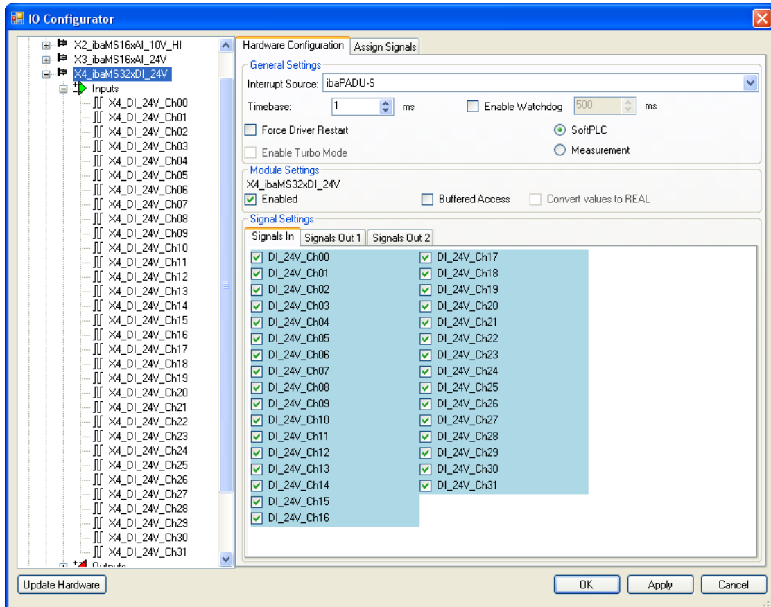
Рис. 14: Входы ibaMS32xDI-24V
