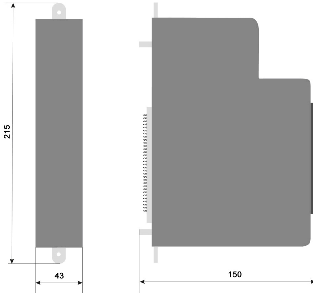
Рис. 19: Размеры модуля (в мм)
