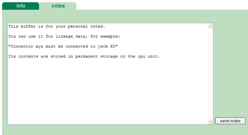
Рис. 10: Вкладка „notes“
