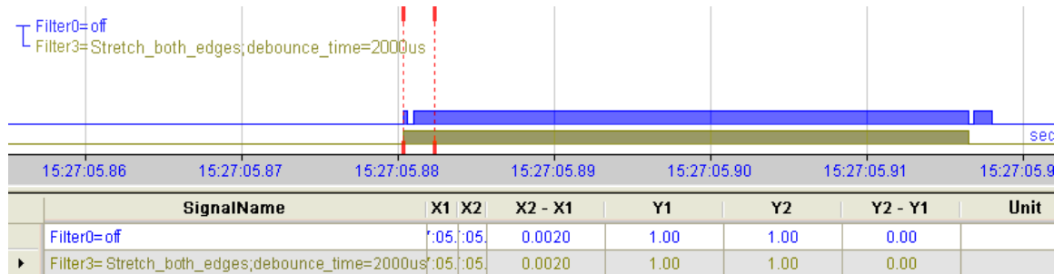
Рис. 5: Фильтр дребезга: "Растянуть оба фронта"
