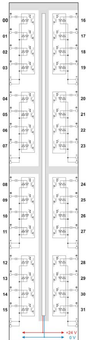
Рис. 2: Схема соединений
