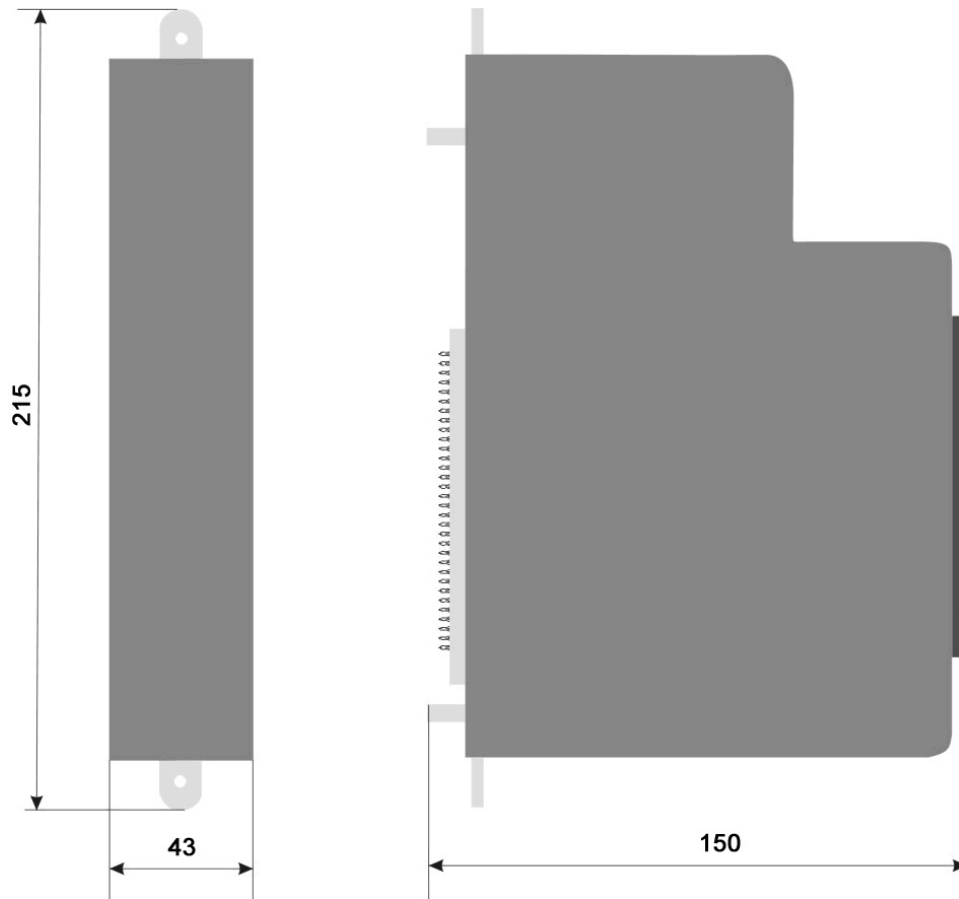
Рис. 17: Размеры модуля (в мм)
