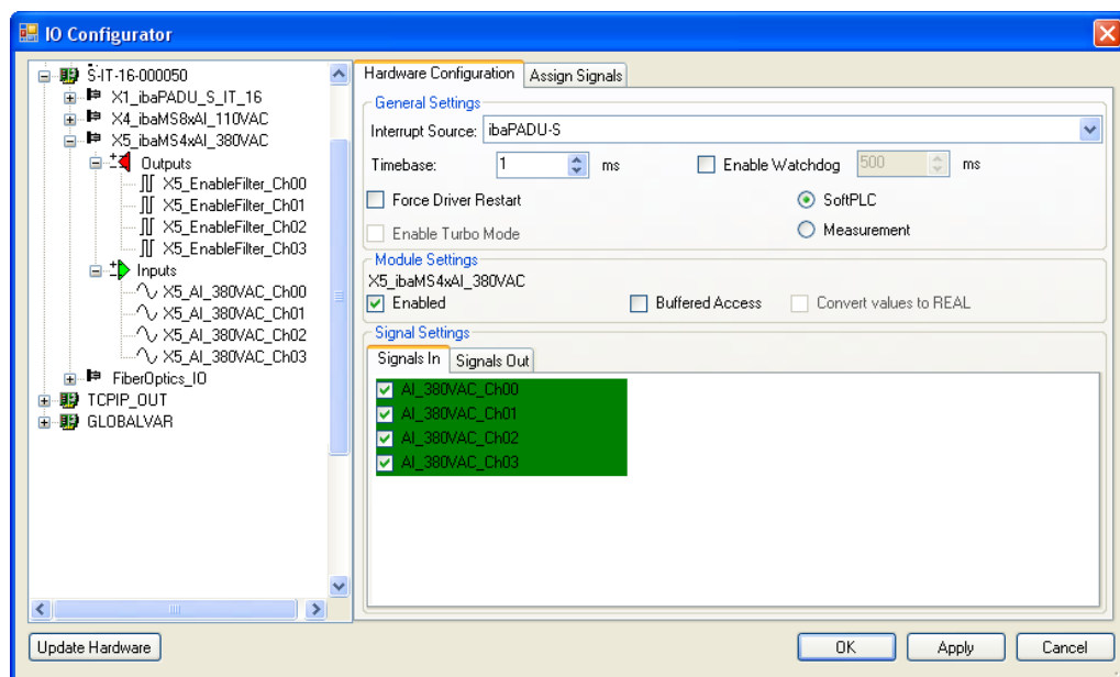
Рис. 12: Входы ibaMS4xAI-380VAC
