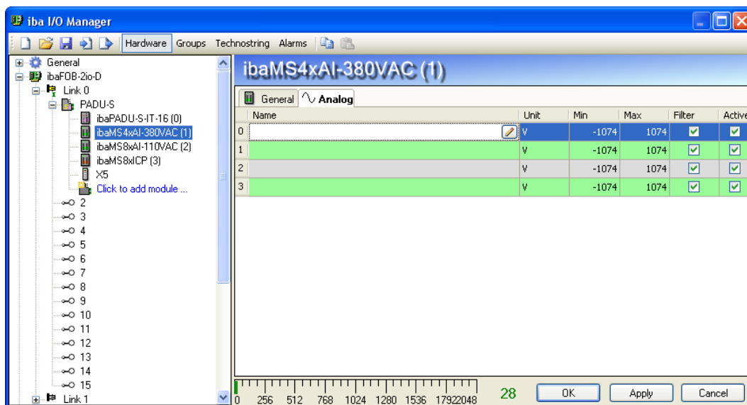
Рис. 11: Диспетчер ввода-вывода, ibaMS4xAI-380VAC – вкладка "Аналоговые"
