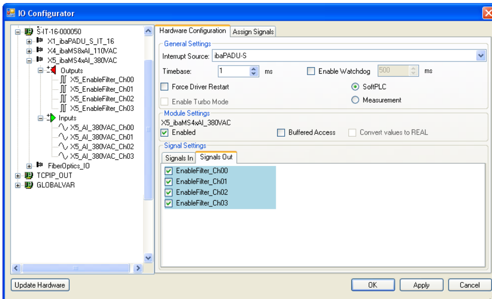
Рис. 13: Выходы ibaMS4xAI-380VAC
