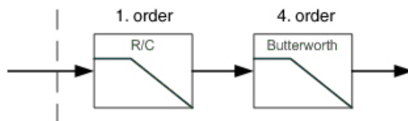
Рис. 3: Секции фильтра
